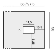
con scatola elettrica with flush mounting box
