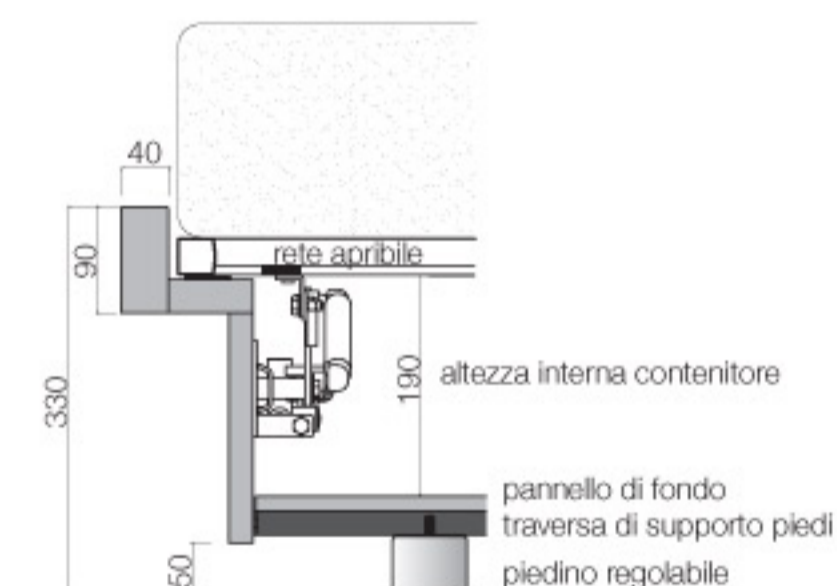
Sezione giroletto H 90 con CONTENITORE
