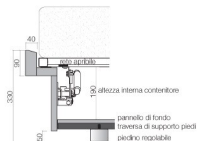
Sezione giroletto H 90 con CONTENITORE
