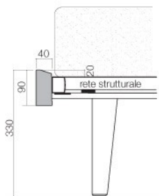
Sezione giroletto H 90 con PIEDE LEGNO
